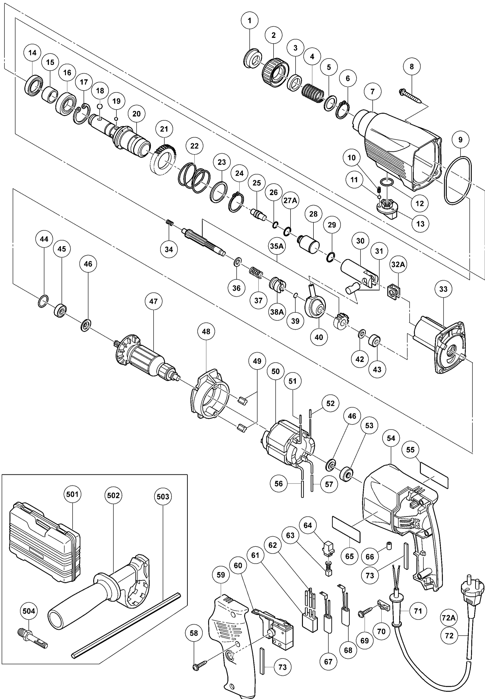
形名 DH24PB
